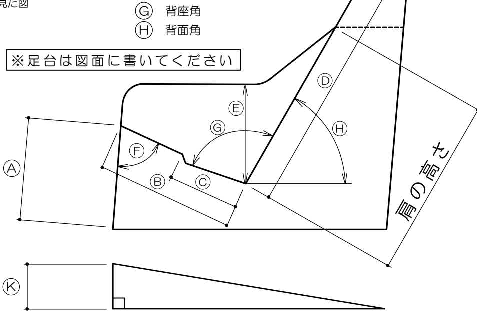
<側面図> 横から見た図
